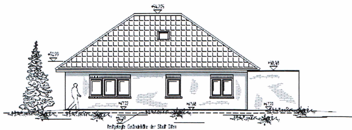
Rückansicht
