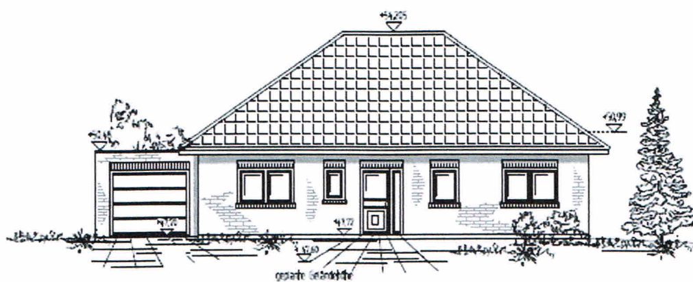
Vorderansicht
