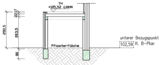
Schnitt B-B
