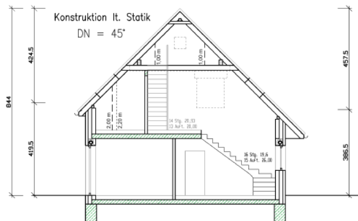
Schnitt A-A
