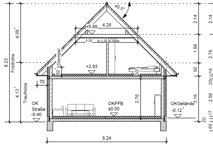
SCHNITT 1 - 1
