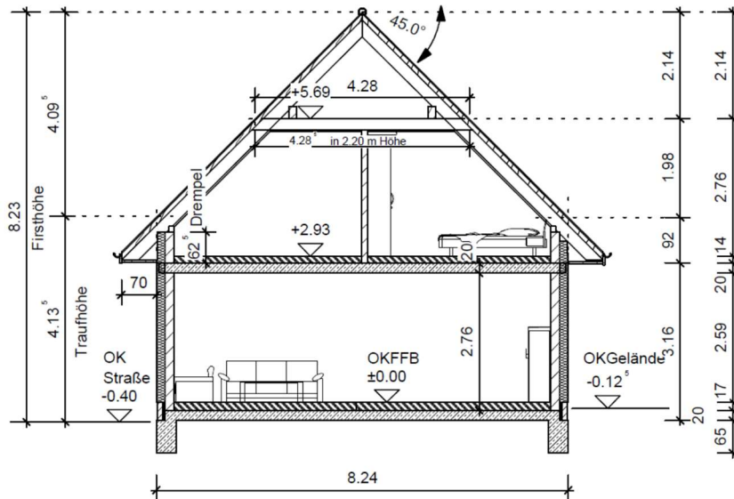
SCHNITT 1 - 1
